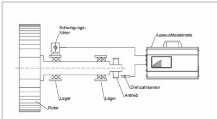
1-Ebenen-Auswuchten
