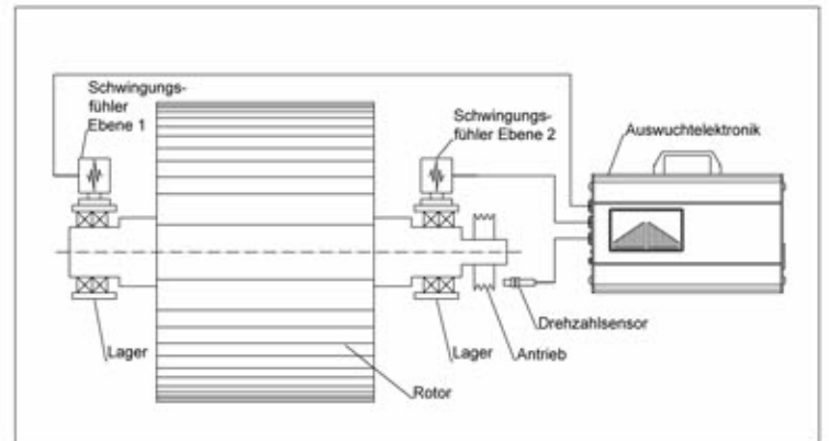
1+ 2-Ebenen-Auswuchten
